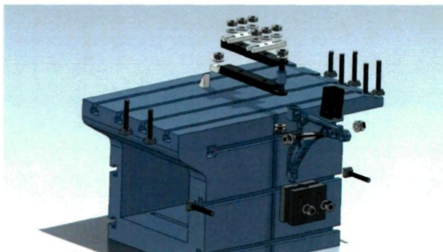
Figure 4.19 : Vue éclatée du montage.
