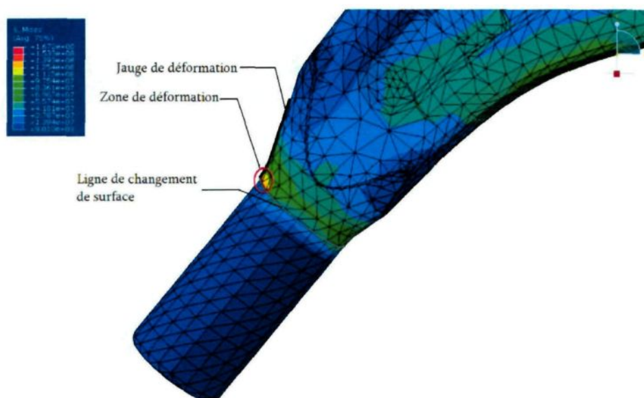
Figure 5.5 : Emplacement jauge N°3 sur le bras de suspension.
