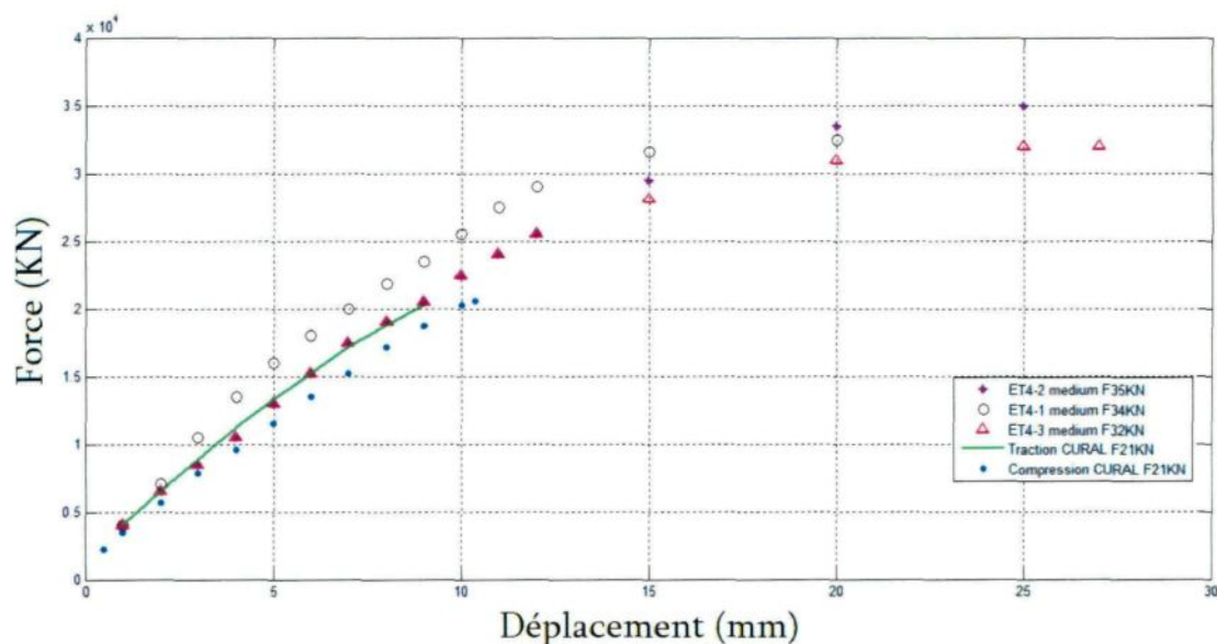
Figure 5.8 : Comparaison courbes de traction et de compression.
