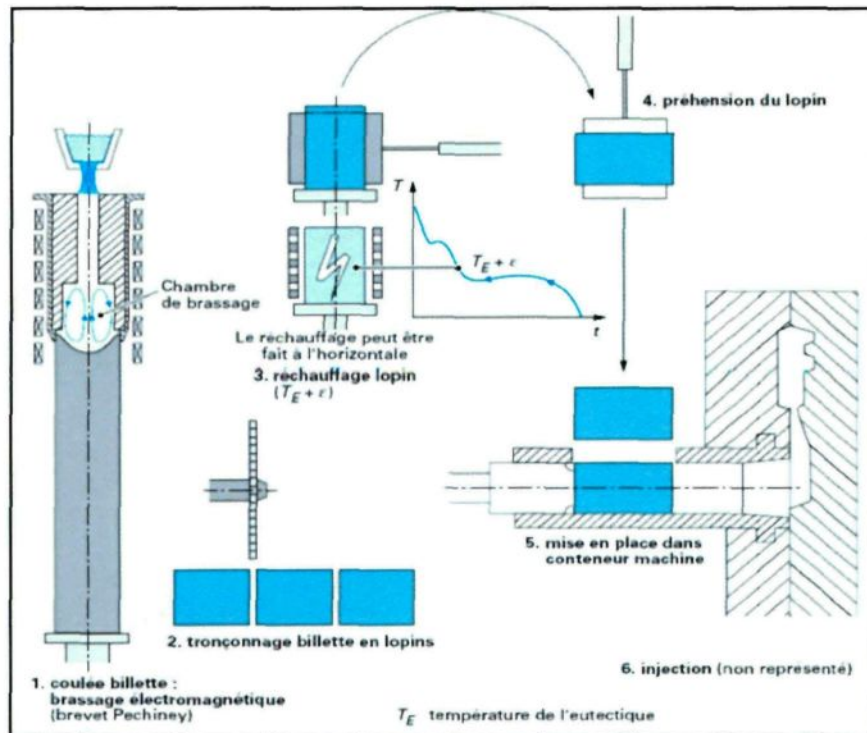
Figure 2.6 : Schéma du principe du thixomoulage [6].
