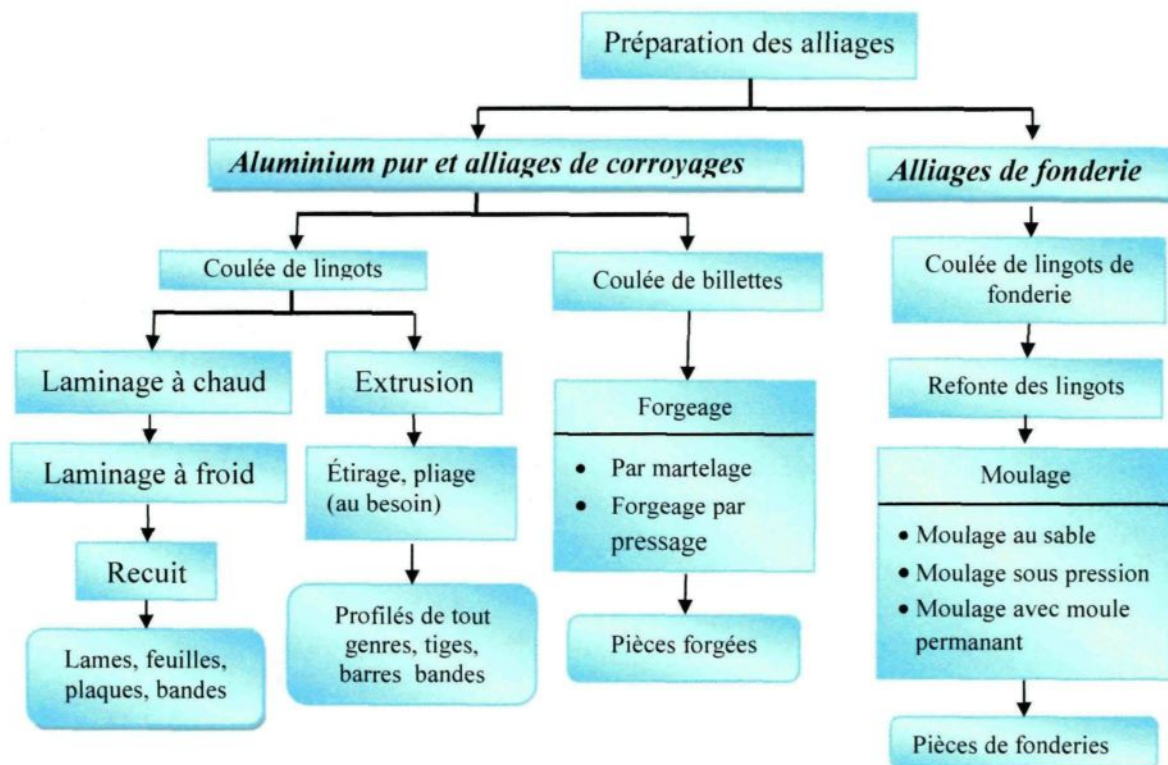
Figure 2.1 : Procédés de transformation de l'aluminium [4].
