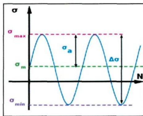
Figure 2.17 : Contraintes alternées dissymétriques -1 < R\sigma < 0 .
