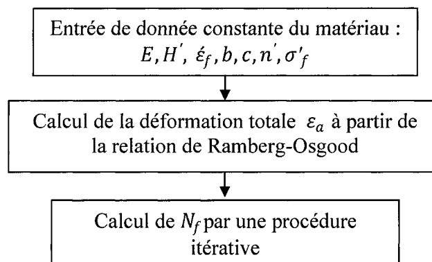
Figure 3.3 : Organigramme des étapes de calcul de la durée de vie.
