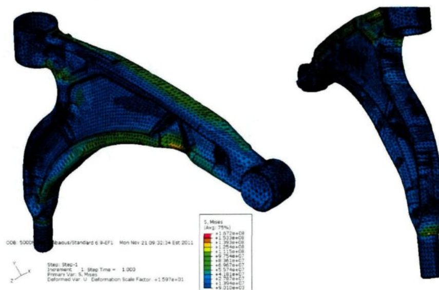
Figure 4.12 : Contrainte maximale pour une force de 5000 N.
