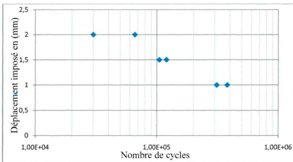
Figure 5.13 : Nombre de cycles expérimental versus le déplacement du bras de suspension.
