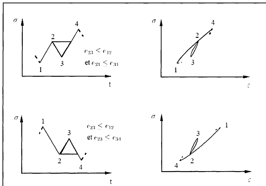
Figure 2.14 : Principe du comptage de cycles Rainflow [19].
