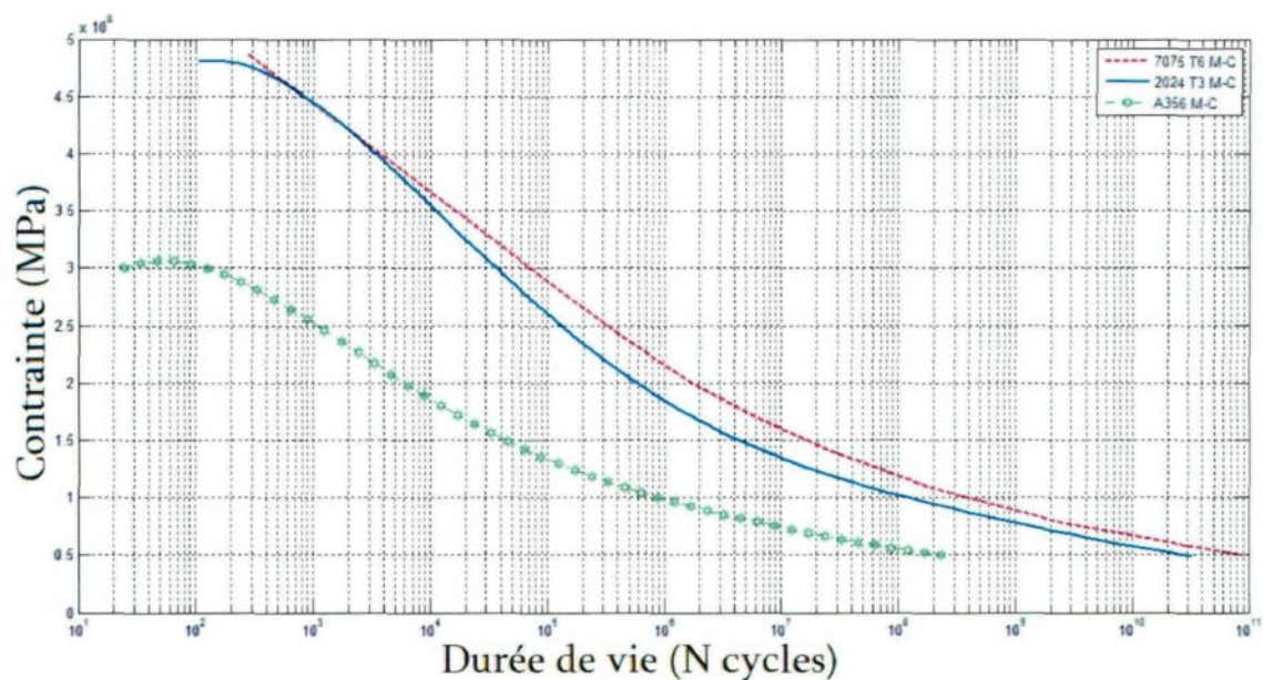
Figure 3.5 : Courbe S-N des alliages 2024 T3, A357 et le 7075 T6 pour la méthode Manson-Coffin.
