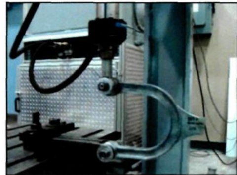
Figure 5.2 : Bras de suspension déformé après le test de traction.
