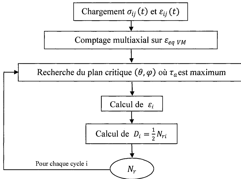
Figure 3.1 : Organigramme du déroulement de la méthode de Wang et Brown.
