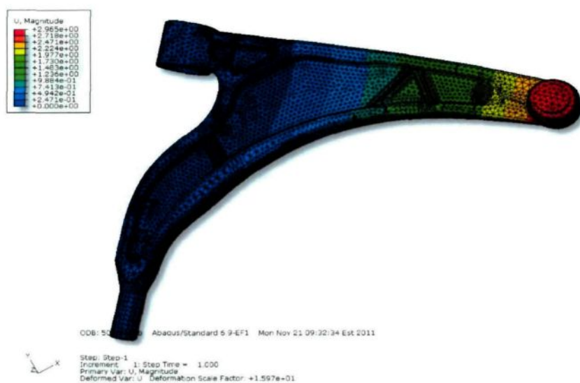
Figure 4.13 : Déplacement maximal pour une force de 5000 N.
