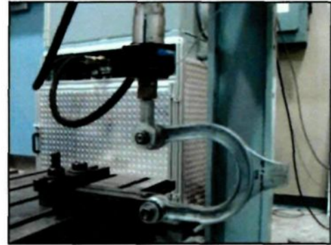
Figure 5.4 : Bras de suspension déformée après le test de compression.
