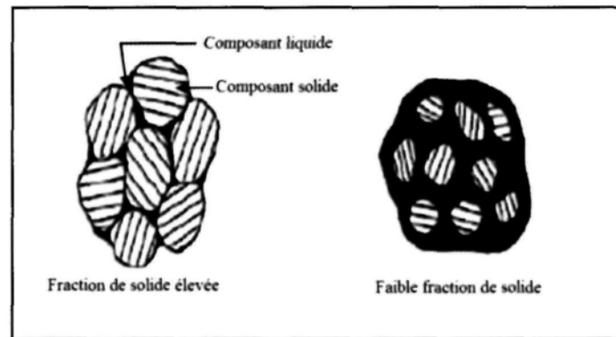
Figure 2.3 : Mécanisme impliqué dans le changement de la morphologie des grains dans la fusion partielle et isotherme (Kiuchi and Kopp, 2002) [8].
