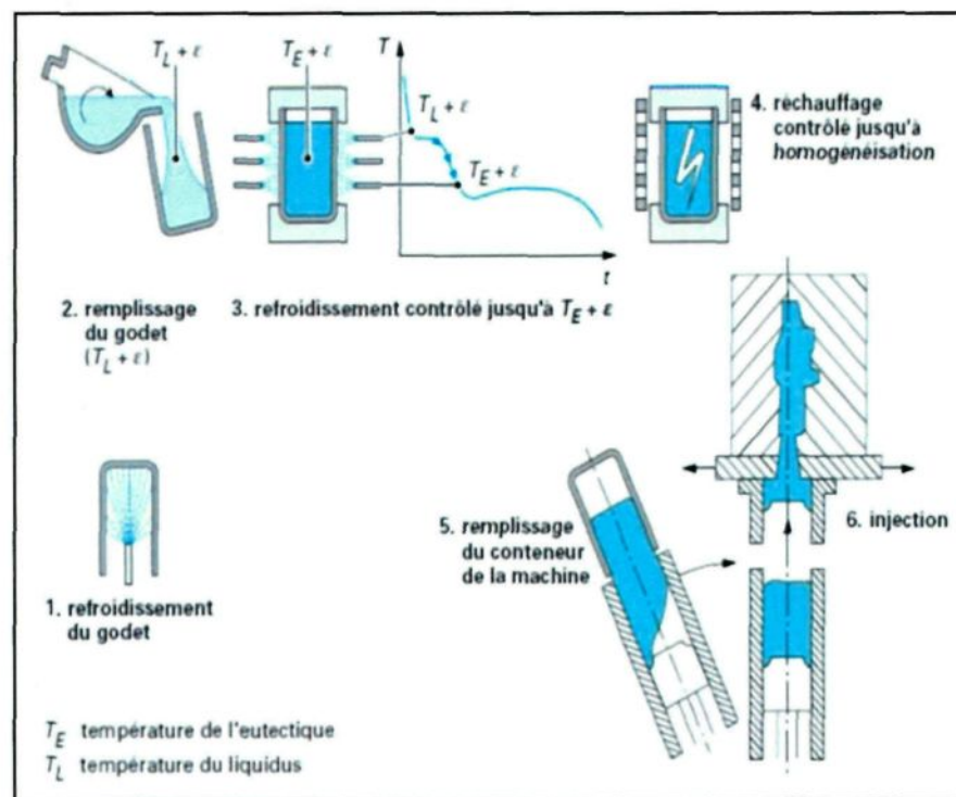
Figure 2.7 : Schéma du principe du rhéomoulage [6].
