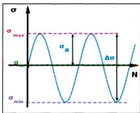
Figure 2.16 : Contraintes alternées symétriques R\sigma = 1 .
