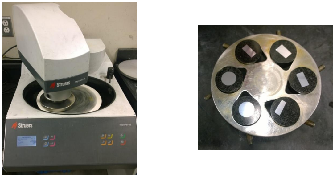
Figure 5.13: Polisseuse et support échantillons (Struers).
