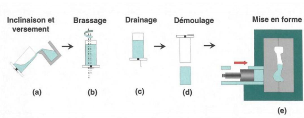
Figure 2.4: Diagramme schématisant le procédé SEED (a-c), et le moulage à haute pression (d-e).
