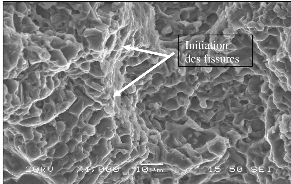
Figure 6.11: Micrographie avec MEB montre le mécanisme de fracture et initiation de fissures de l'alliage A357-T6 semi-solide après test de fatigue.
