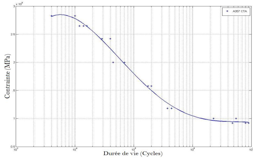
Figure 4.1 : Courbe S-N pour des éprouvettes en aluminium A357 Semi-solide.
