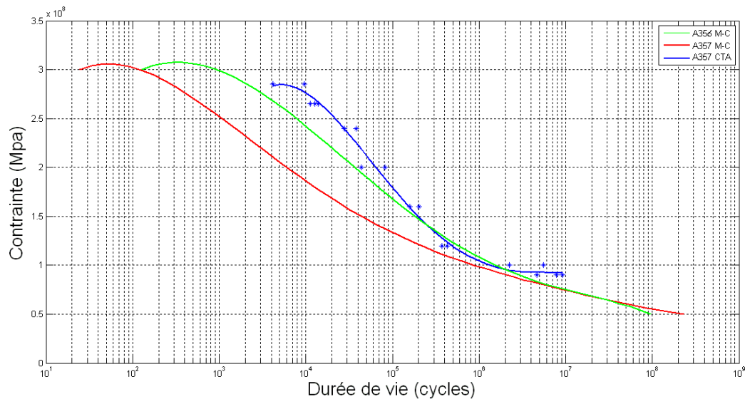
Figure 4.4 : Courbe S-N de l'aluminium A357 SS après correction des coefficients sigma et b versus la courbe expérimentale.
